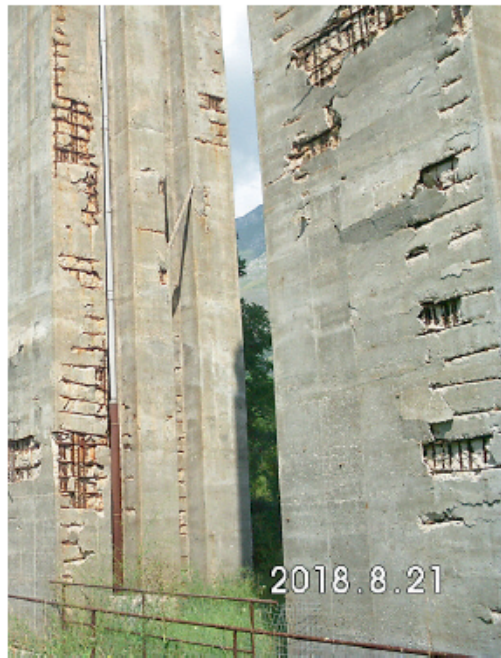
Lo stato in cui versano i piloni che sostengono il viadotto di Assergi dell'autostrada A24. Le due foto sono state scattate martedì scorso
